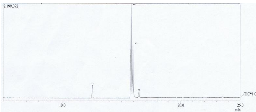
Gambar 2. Kromatogram Hasil GC-MS Minyak Biji Bunga Matahari
