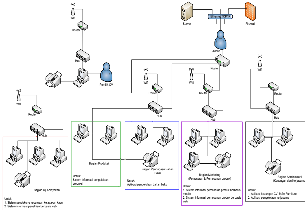
Gambar 5. Topologi Jaringan
