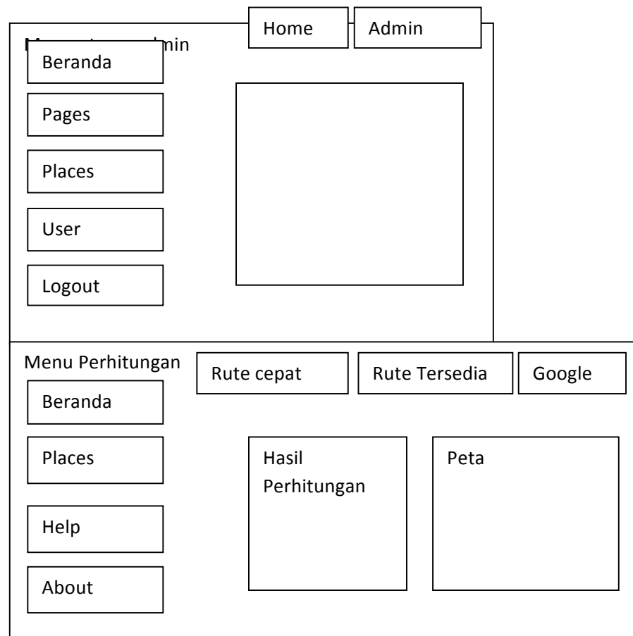
Gambar 4.10. Rancangan Menu Perhitungan
