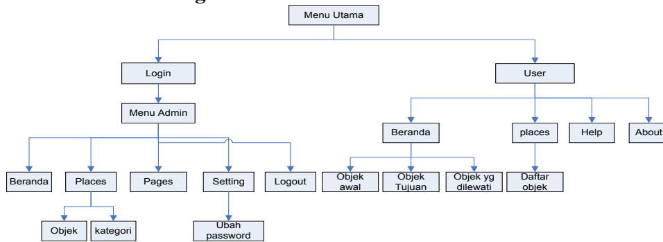
Gambar 4.8 Rancangan Form Menu Utama
