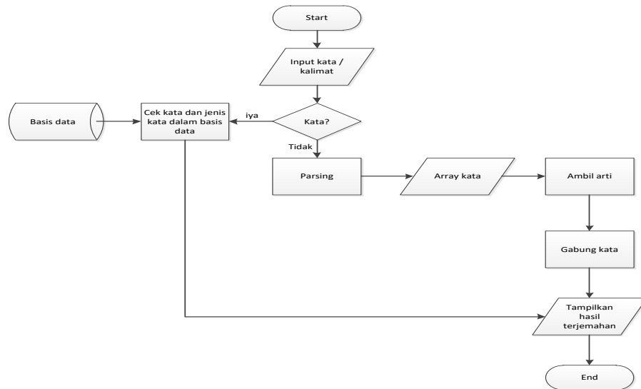
Gambar 3.: Flowchart penerjemahan
