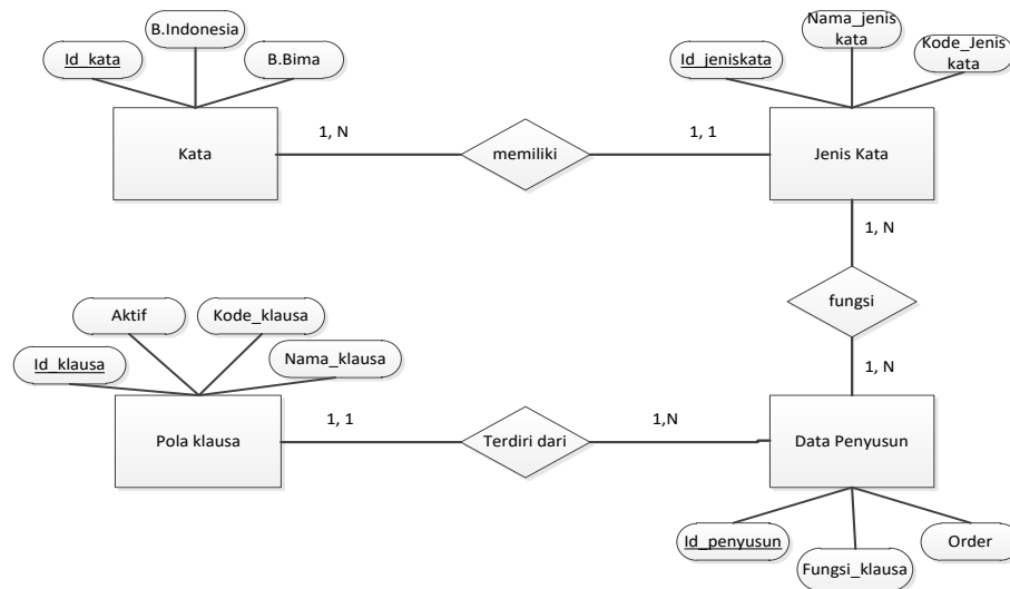
Gambar 4.: ERD Kamus
