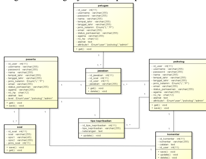
Gambar 4. Class Diagram Tes Kepribadian
