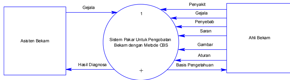
Gambar 4 : Perancangan Diagram Kontek
