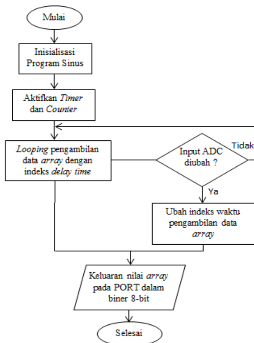
Gambar 3. Diagram alir program pembangkit gelombang sinus
