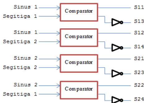
Gambar 5. Diagram blok komparator
