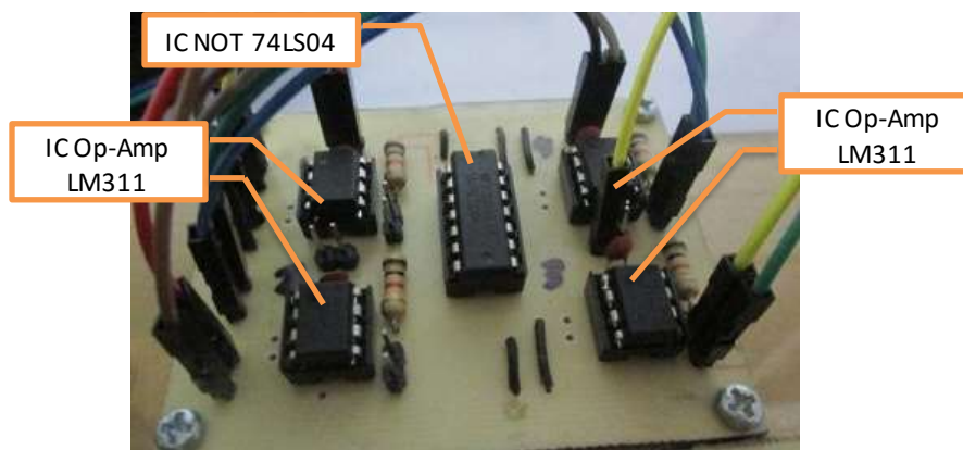
Gambar 11. Rangkaian perbandingan dengan Op-Amp LM311 dan IC NOT 74LS04
