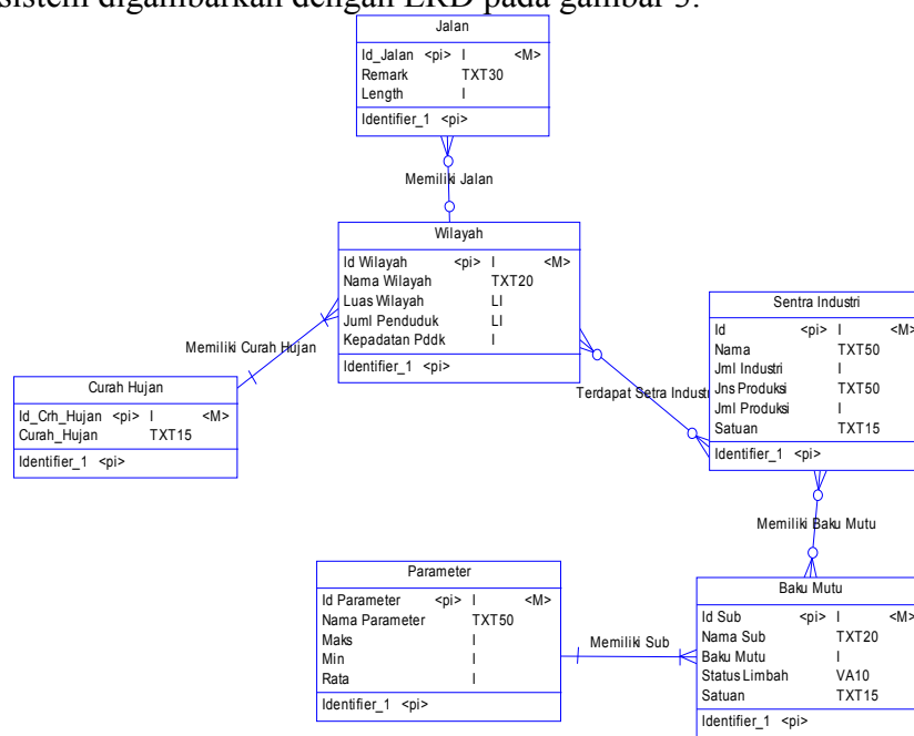
Gambar 3. ERD Sistem
