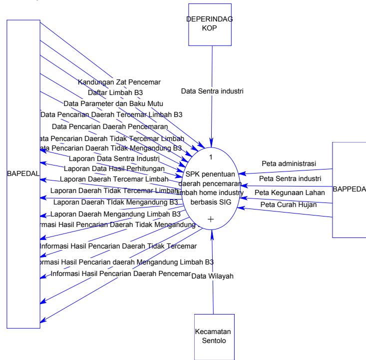
Gambar 1. Diagram konteks
