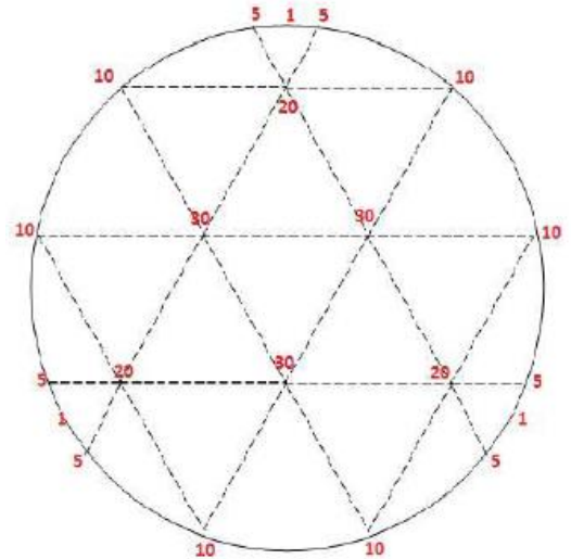
Gambar 8. Koefisien trinomial pangkat 5 pada lingkaran.
