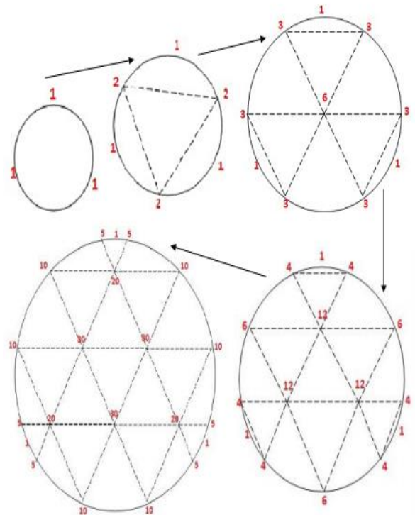
Gambar 9. Koefisien-koefisien trinomial pada lingkaran.
